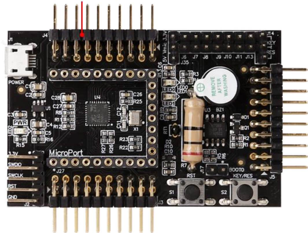
图 7.1 AM116-Core MiniPort
