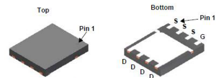
PQFN8 5x6 (Power 56) CASE 483AF
