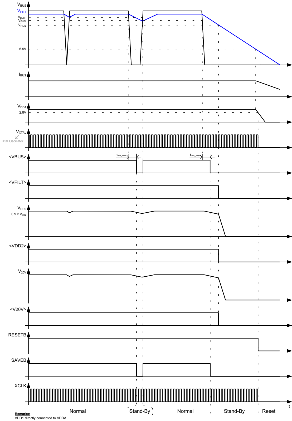
图 15. 关断行为
