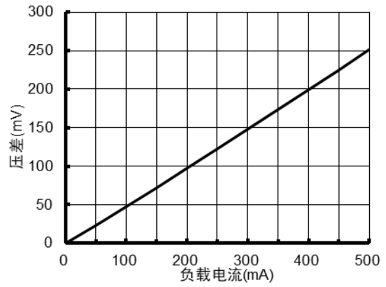
图 2.3 压差与负载电流的关系
