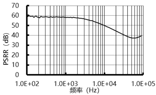
图 2.10 PSRR 与频率的关系 ( I_{\text{out}}=1\text{mA} )
