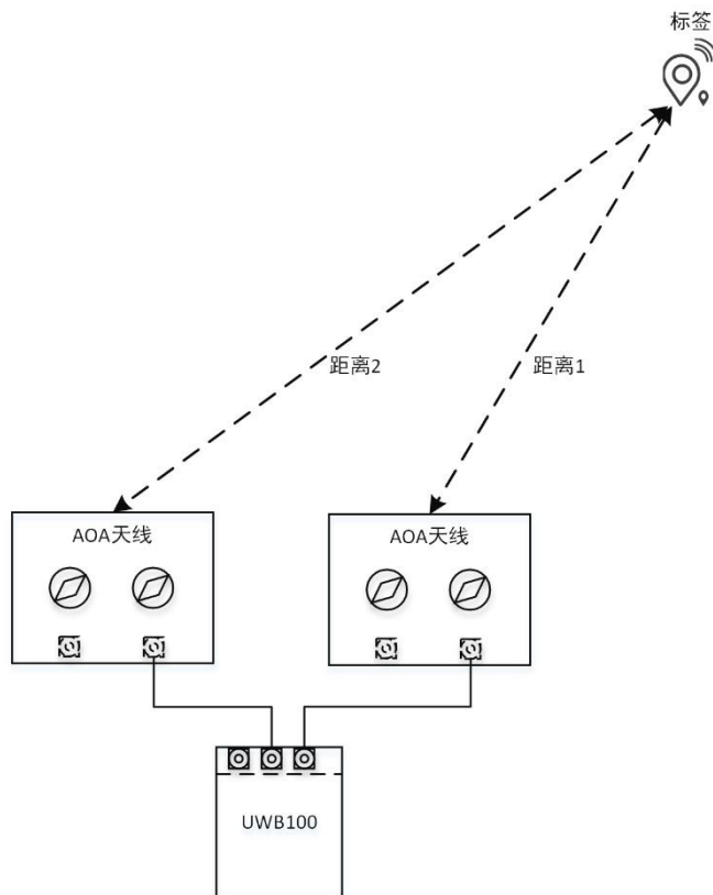
图 2.2 双路 TOF 测距示意
