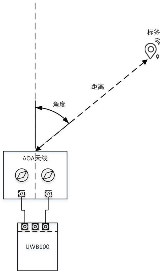
图 2.3 2D AOA 测距示意
