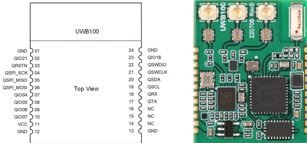
图 1.1 UWB100 模块引脚
