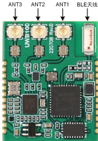
图 1.2 天线定义
