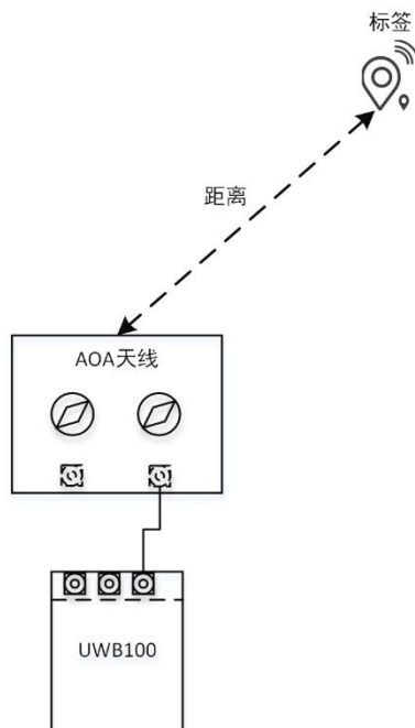
图 2.1 单路 TOF 测距示意
